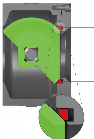
Valvola Schubert & Salzer a settore sferico
