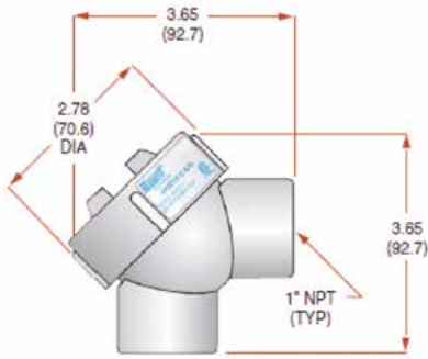
Conduit elbow style Model B220-873 & B220-874
